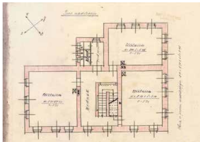
Tloris nadstropja grahovske šole, Šolski list, 1929–1936, hrani SŠM.
